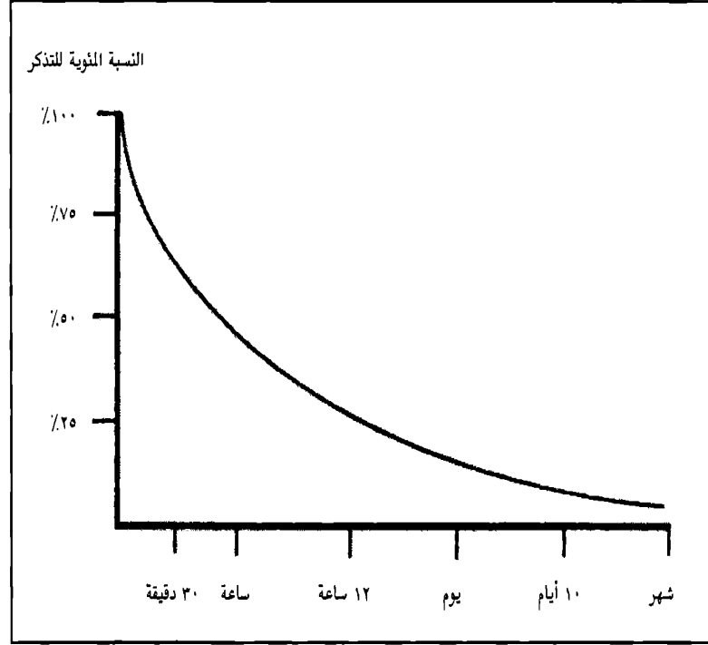
الشكل رقم ٢ منحنى إينجهاس
